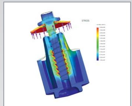
Setzsimulation I
