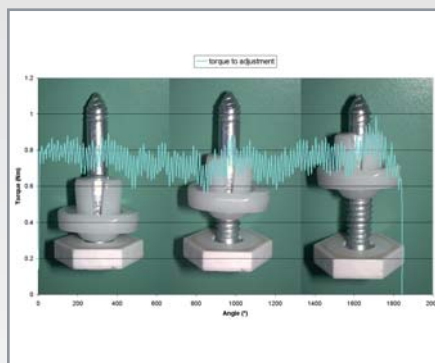
Setzverlauf beim Eindrehmoment
