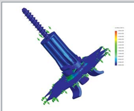
Simulation einer Sonderbefestigung für die weiße Ware
