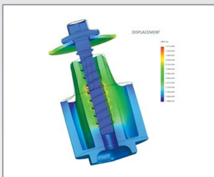
Setzsimulation II
