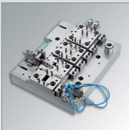
Folgeverbundwerkzeug
